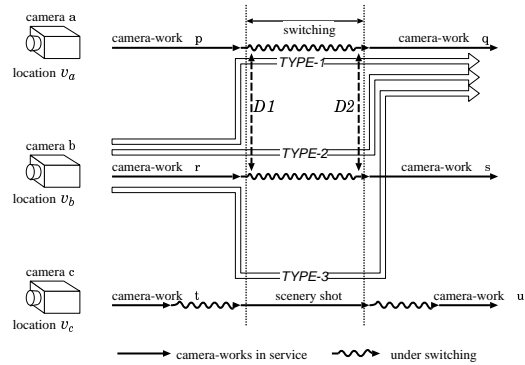
図 4 映像切替えの経路 Fig.4 Pathes on video switching.
