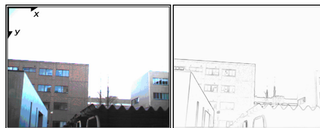
図 5：PDA カメラ画像（左）と輝度変化の二乗和を求めた結果画像（右）
