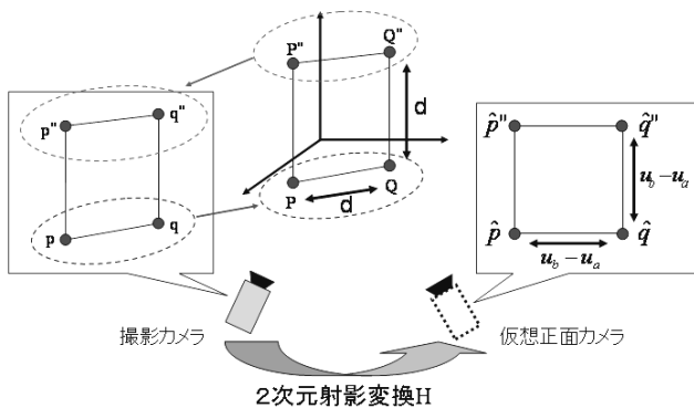
図 4 : 撮影画像と形状平面間の 2次元射影変換の推定
